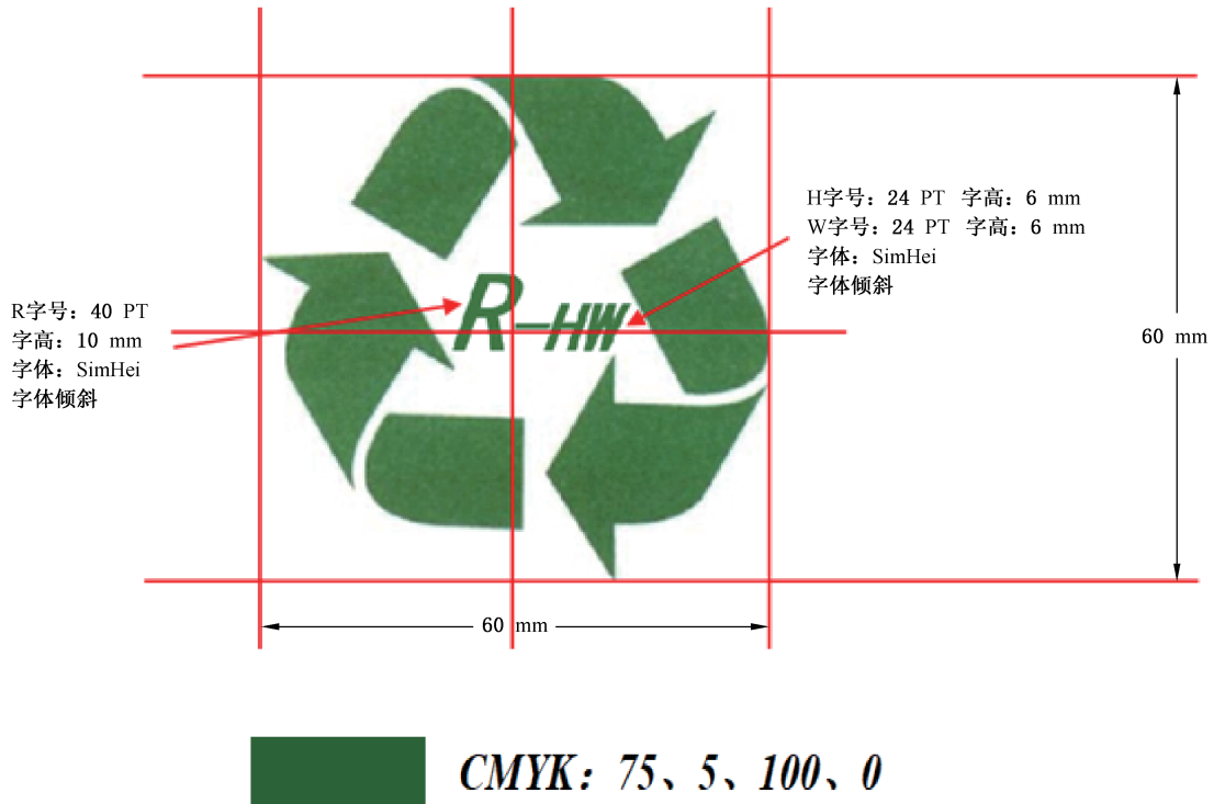
图 A.1 危险废物综合利用产物标识样式及尺寸
